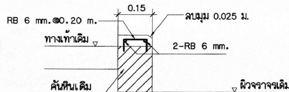
แบบก่อสร้างเสริมคันทัน คสล.
