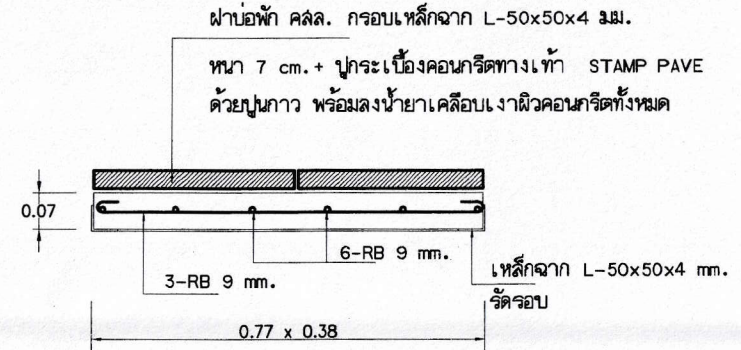
รูปด้าน ฝาบ่อพัก ค.ส.ล.
