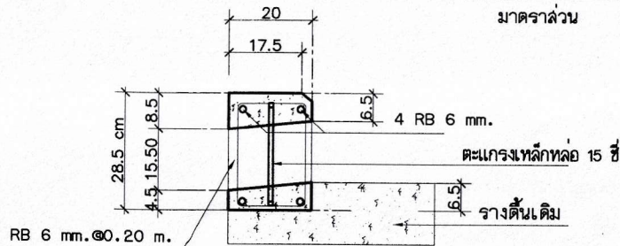
แบบเสริมเหล็กคันทัน รางต้น
