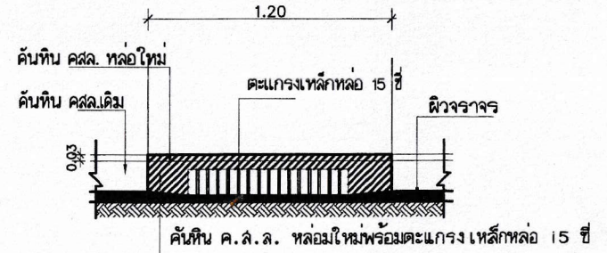
รูปด้านหน้า ช่องตะแกรงรับน้ำ
