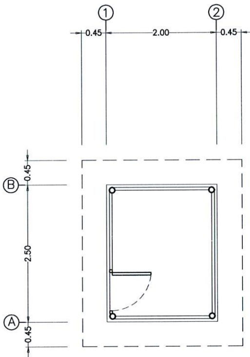
แปลนพื้นห้องเก็บปั้มน้ำ มาตราส่วน 1 : 50
