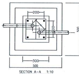
SECTION A-A 1:10
