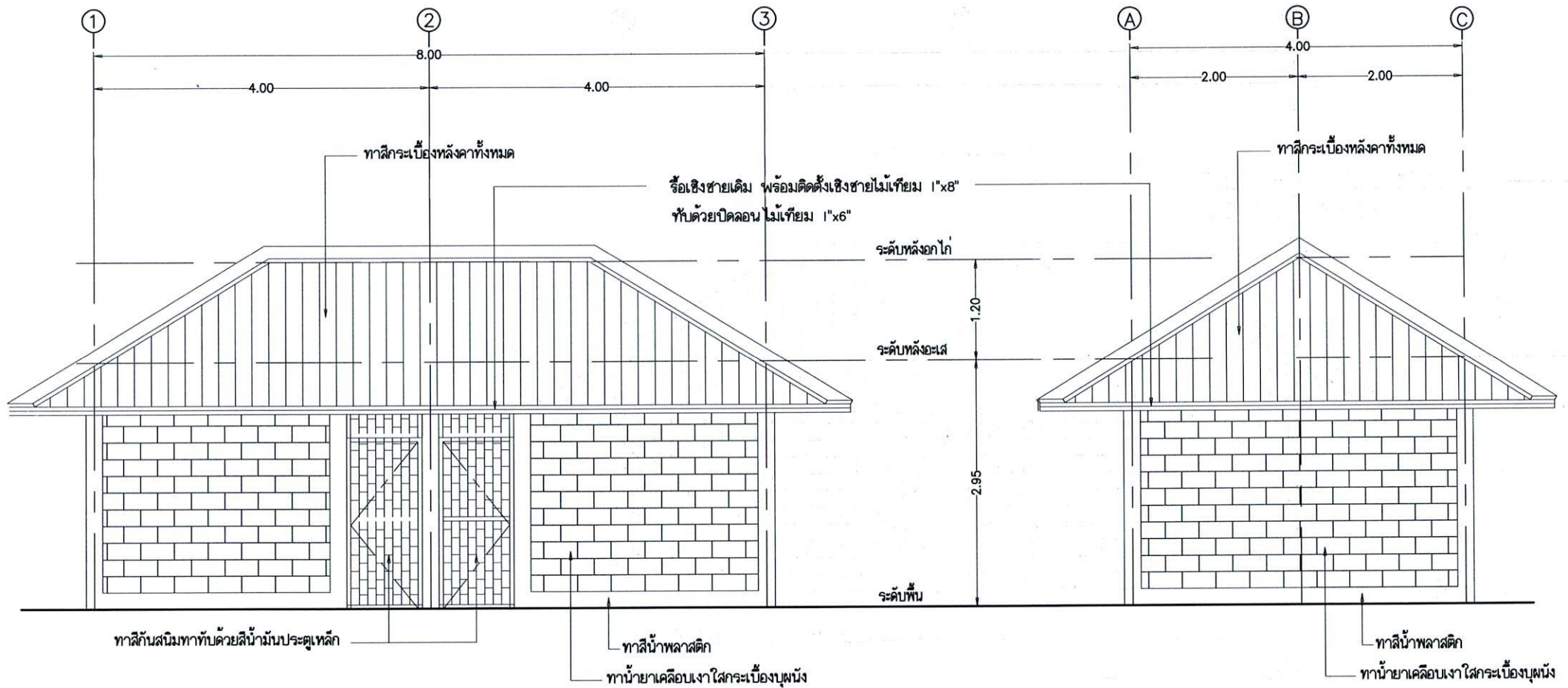
รูปด้านข้างห้องน้ำ มาตราส่วน 1 : 100
