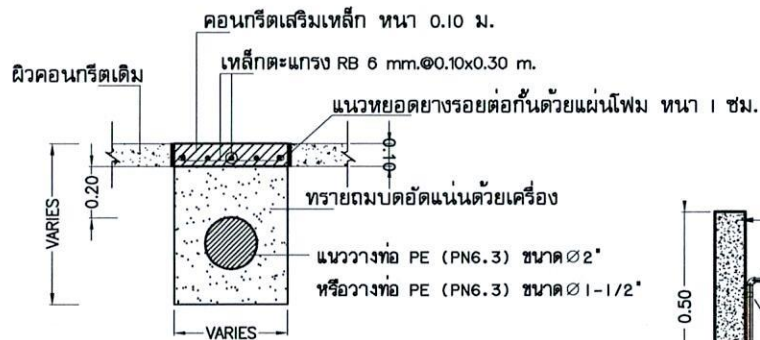
รูปตัดกรณีแนววางท่อ PE ตัดผ่านพื้น ค.ล.ล. เดิม
