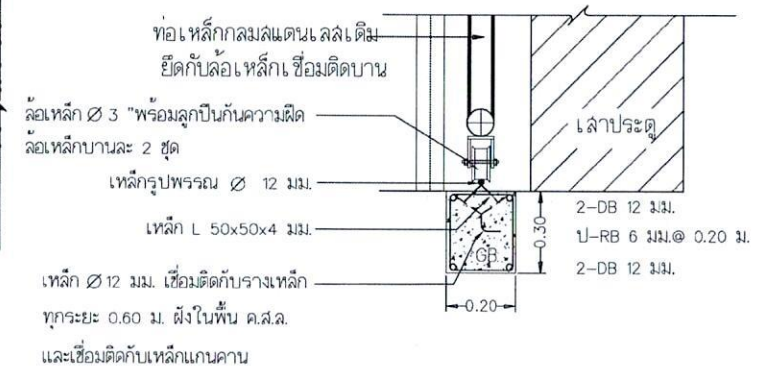
ขยายติดตั้งรางประตูบานเลื่อน มาตราส่วน 1:10
