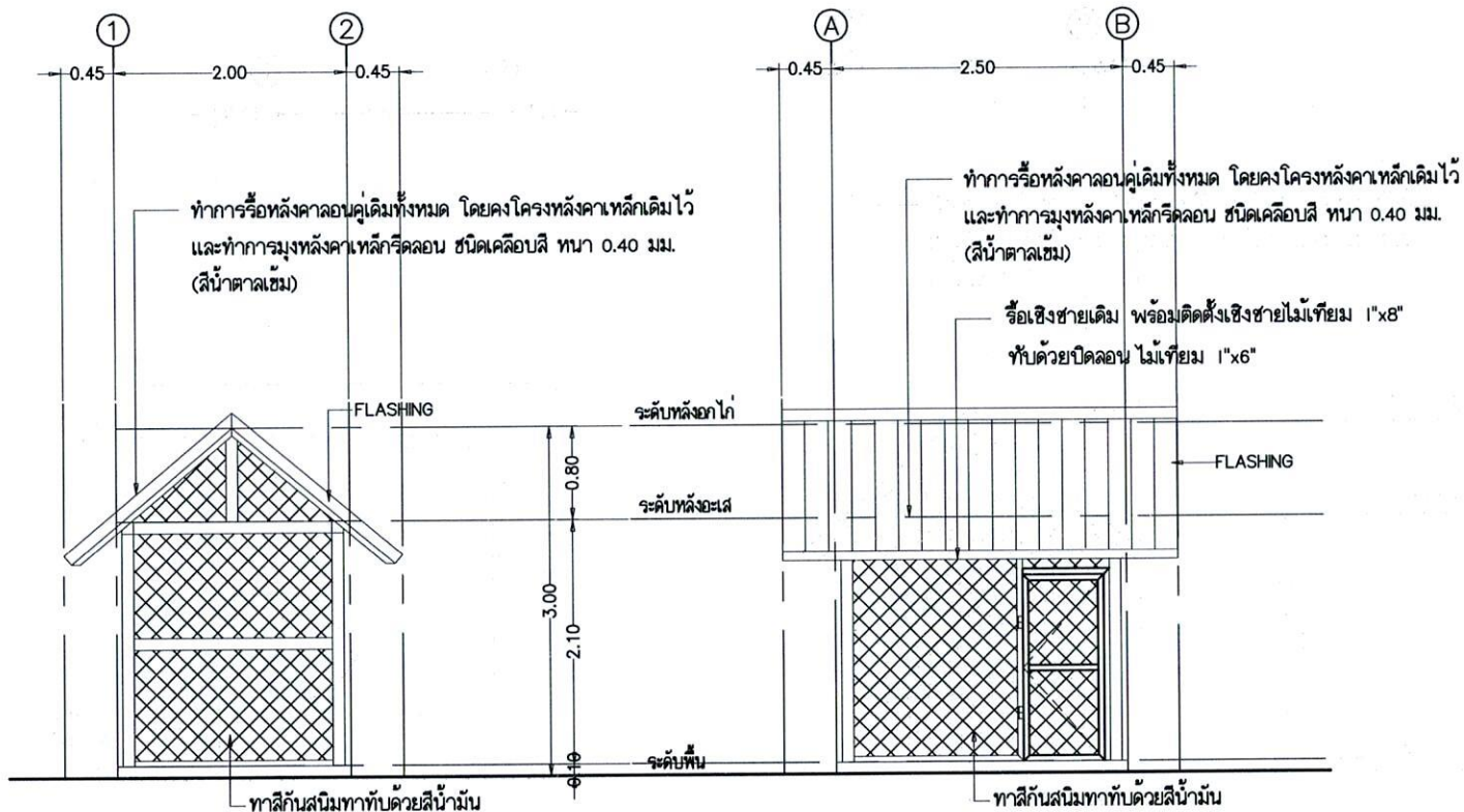
รูปด้านข้างห้องเก็บปั้มน้ำ มาตราส่วน 1 : 50
