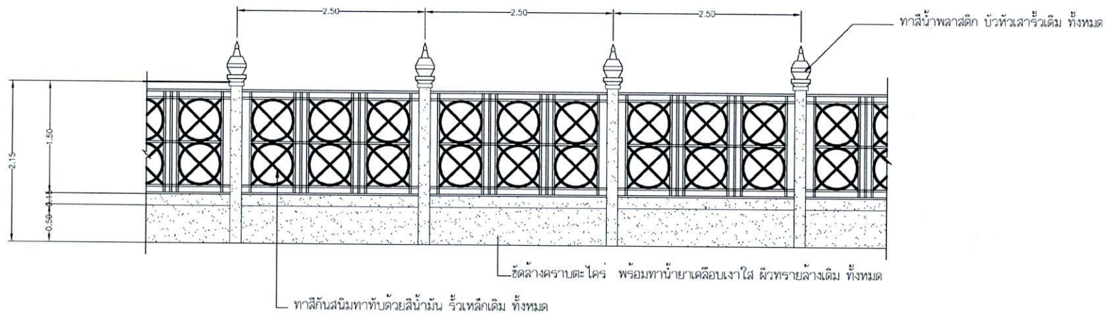
รูปด้านทาสีรั้วด้านหน้า มาตราส่วน 1:50
