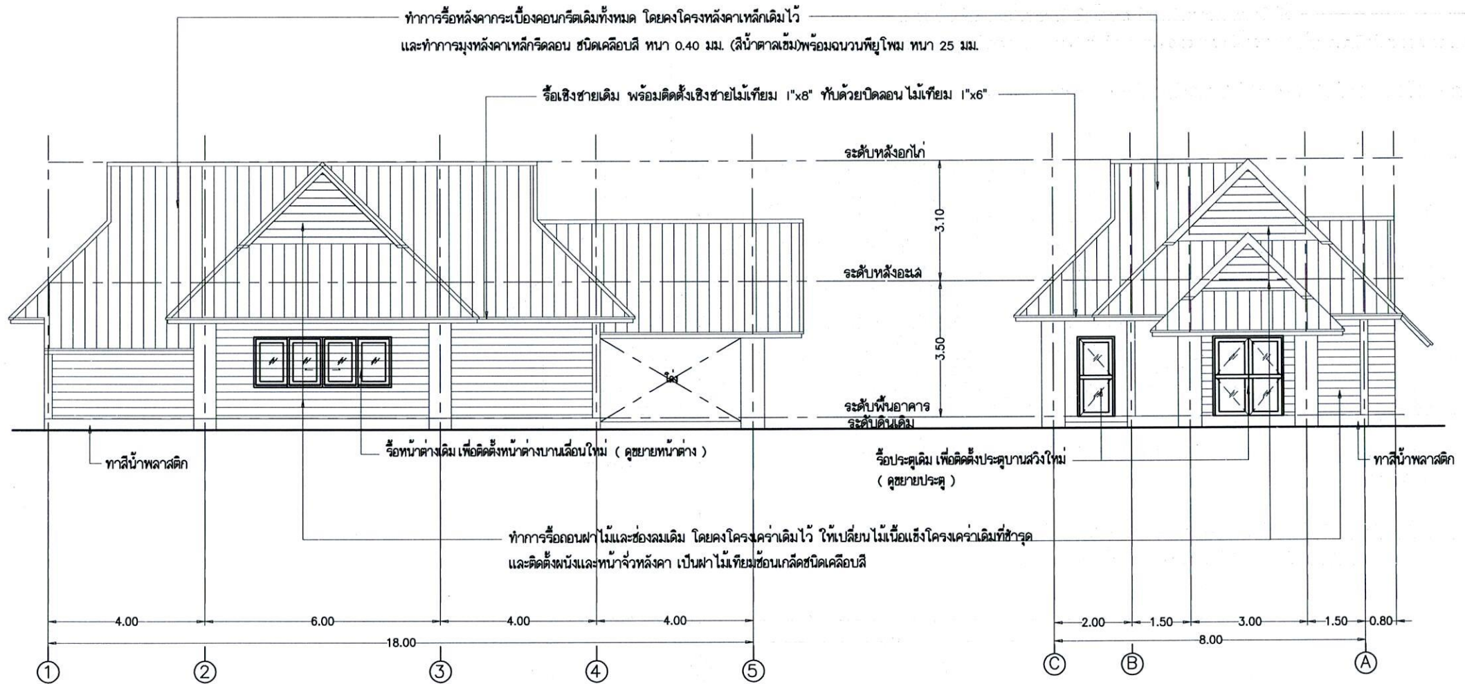
รูปด้านหน้าอาคารที่ทำการ มาตราส่วน 1 : 100
