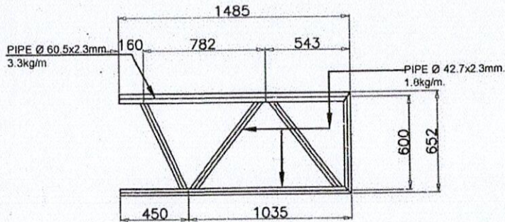
แบบขยาย STRINGER 2
