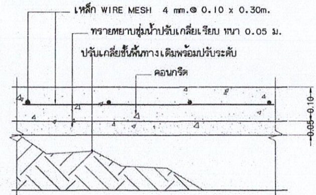
รายละเอียดพื้นคอนกรีตเสริมเหล็ก scale 1:10
