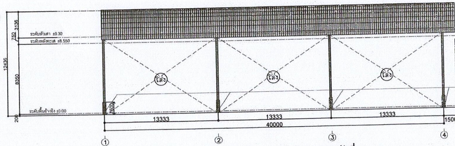
รูปด้านทิศเหนือและทิศใต้ อาคารหลังที่ 3
