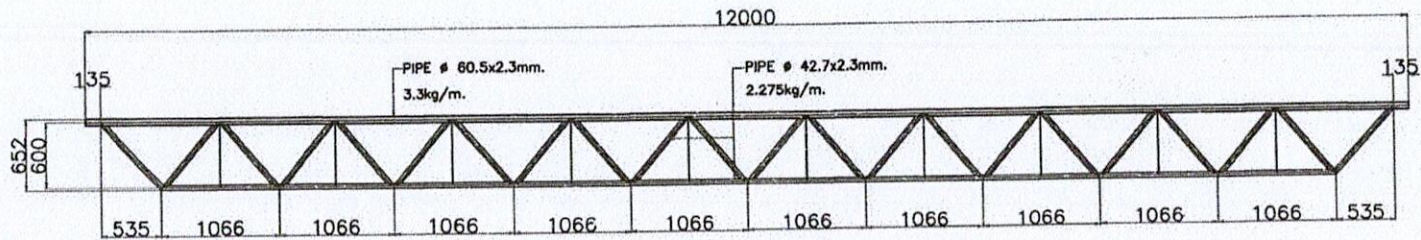
แบบขยาย STRINGER
