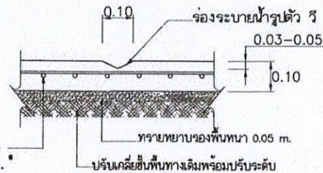
แบบขยายร่องระบายน้ำรูปตัว วี มาตราส่วน 1 : 5
