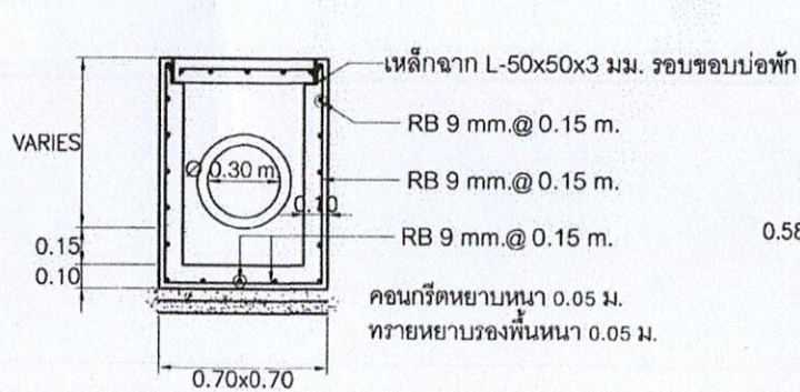
รูปตัดบ่อพัก(B.) คสล. มาตราส่วน 1 : 25
