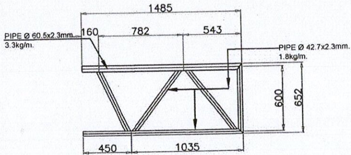
แบบขยาย STRINGER 2
