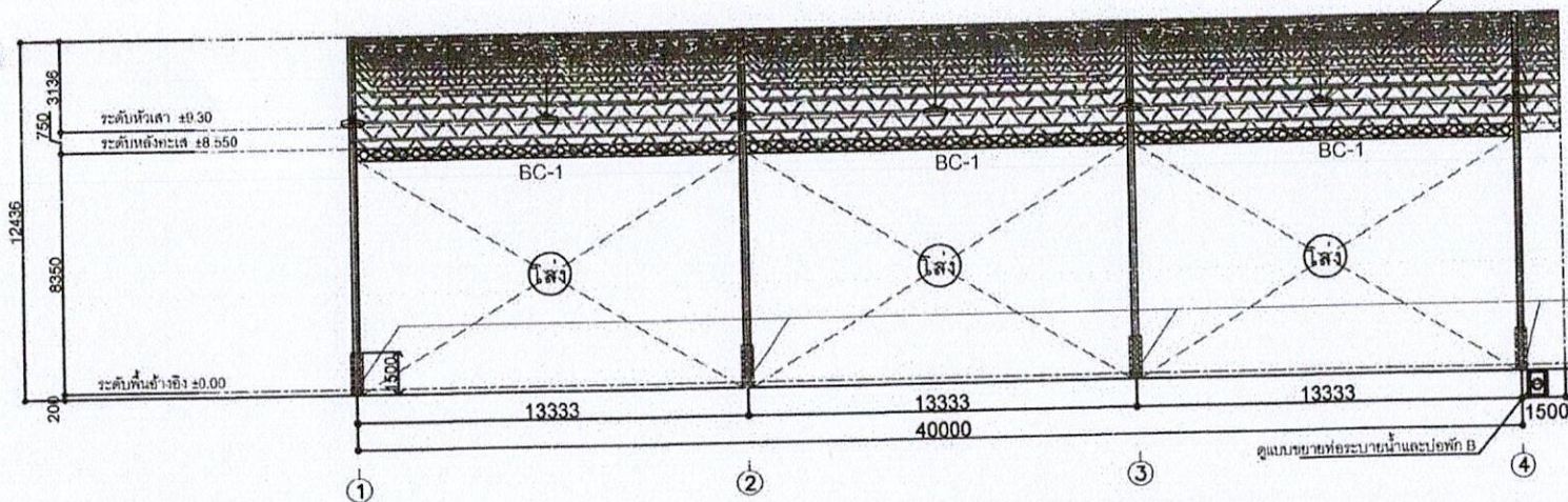
รูปตัด B-B อาคารหลังที่ 3
