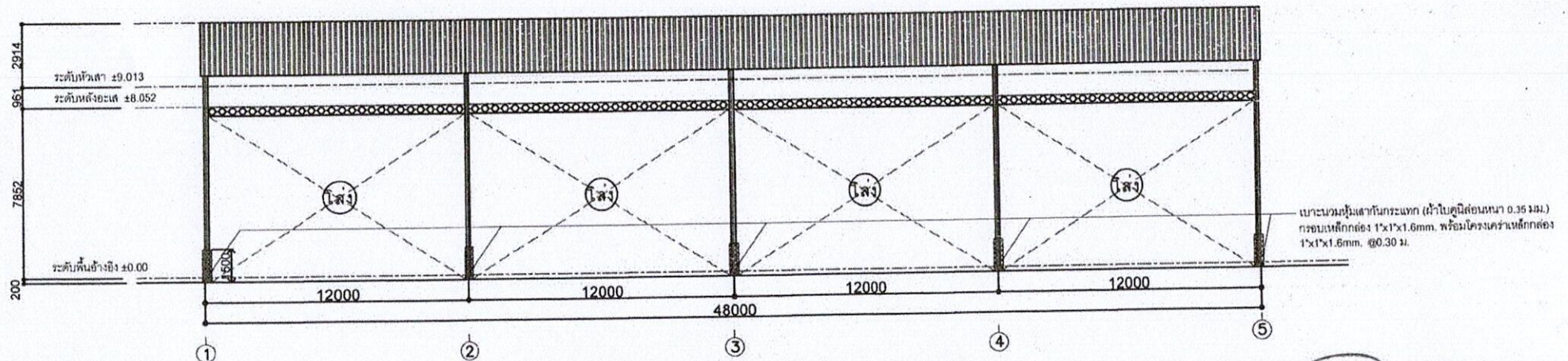
รูปด้านทิศเหนือและทิศใต้ อาคารหลังที่ 2
