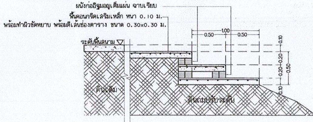
แบบขยายบันได not scale
