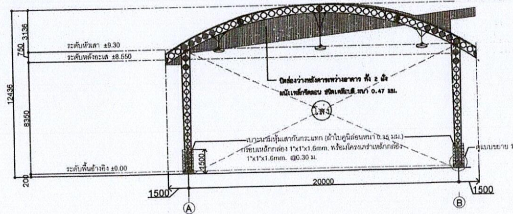
ทิศตะวันออกและทิศตะวันตก อาคารหลังที่ 3
