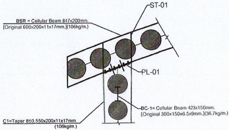
แบบขยาย 3 Scale Not to scale
