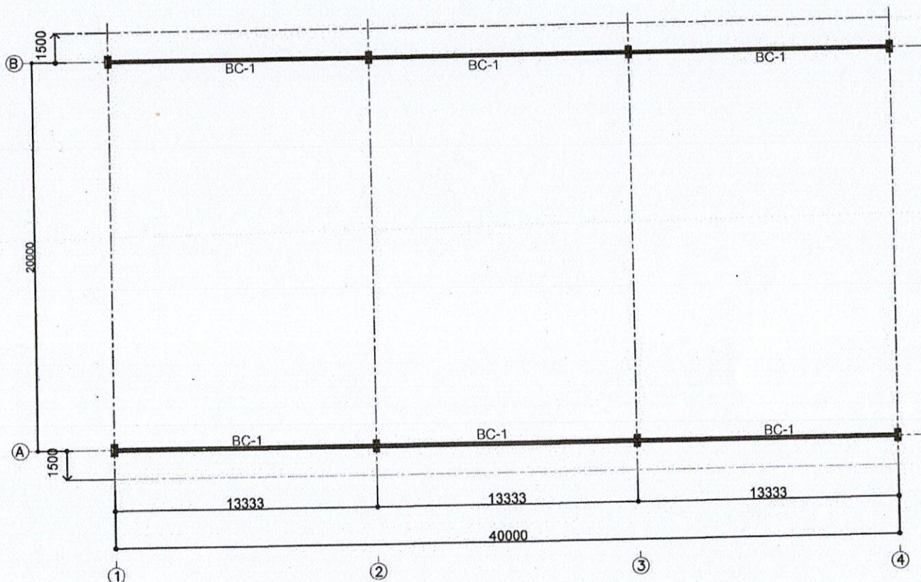
แบบแปลนโครงสร้างคานรัตรอบ อาคารหลังที่ 3
