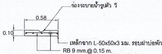
รูปตัดฝาบ่อพัก(B.) คสล. มาตราส่วน 1 : 25
