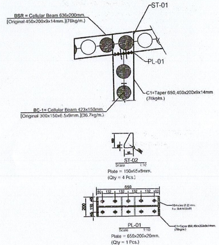
แบบขยาย 3 Scale Not to scale
