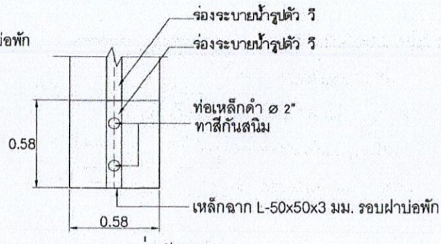
แปลนขยายฝาบ่อพัก(B.) คสล. มาตราส่วน 1 : 25
