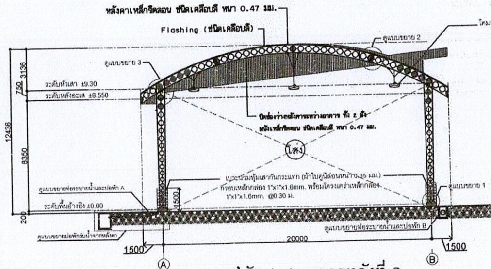
รูปตัด A-A อาคารหลังที่ 3
