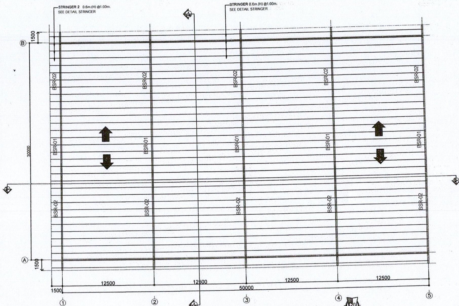
แบบแปลนโครงสร้างหลังคา อาคารหลังที่ 1
