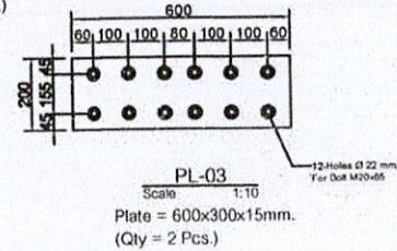
แบบขยาย 2 Scale Not to scale
