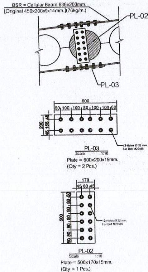
แบบขยาย 2 Scale Not to scale
