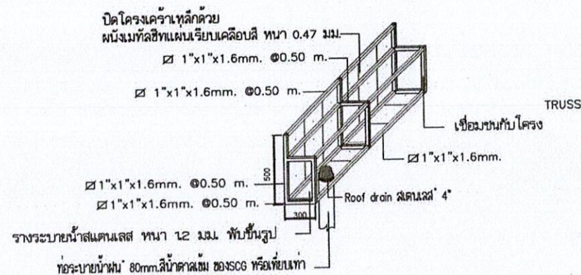
แบบขยาย 4 Scale 1:10
