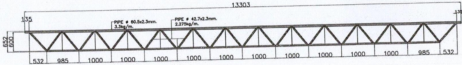
แบบขยาย STRINGER
