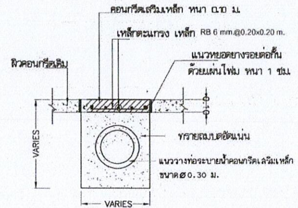
รูปตัดแนววางท่อระบายน้ำ ตัดผ่านพื้น ค.ส.ล.เดิม NOT TO SCALE
