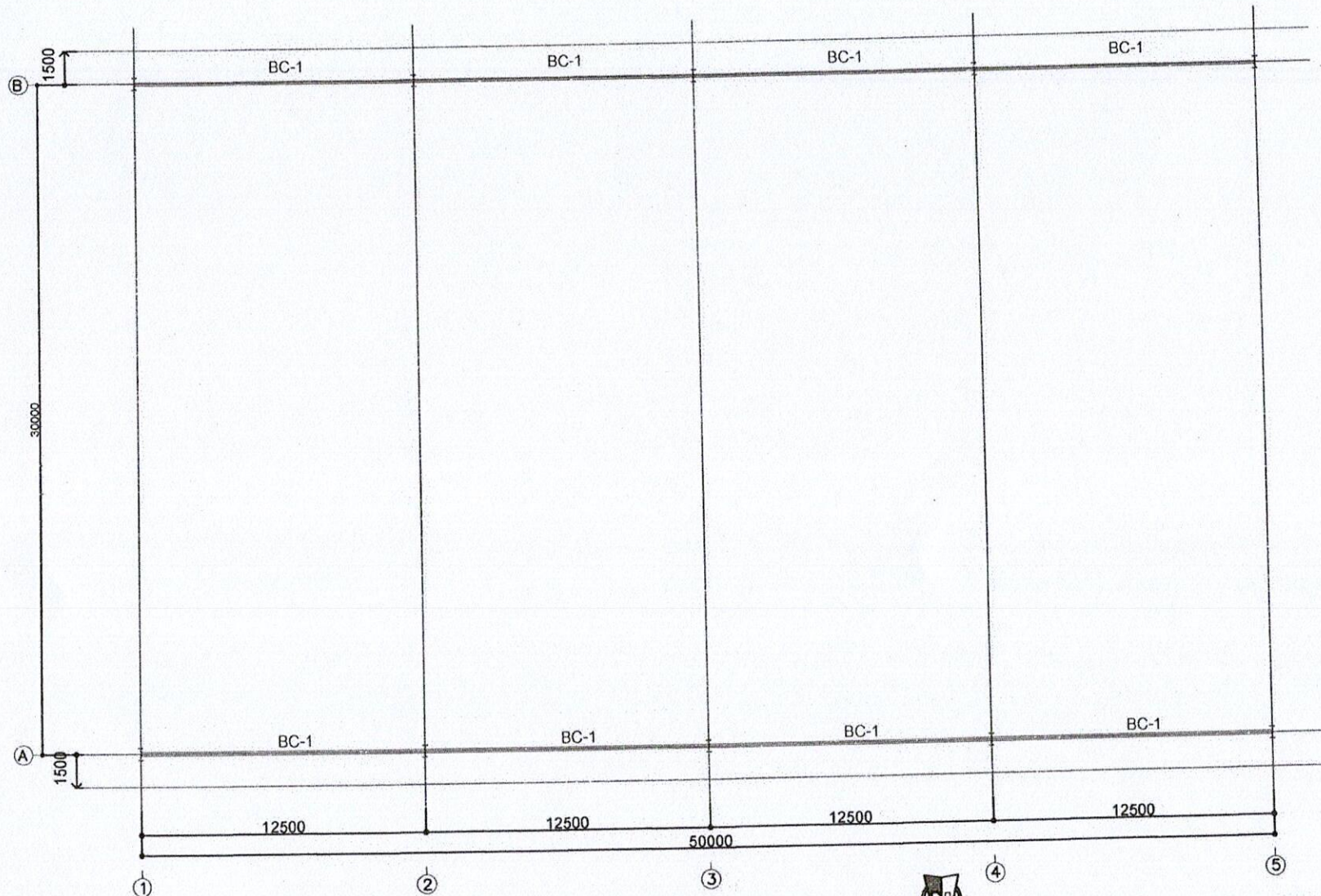
แบบแปลนโครงสร้างคานรัตรอบ อาคารหลังที่ 1
