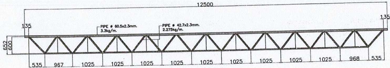
แบบขยาย STRINGER
