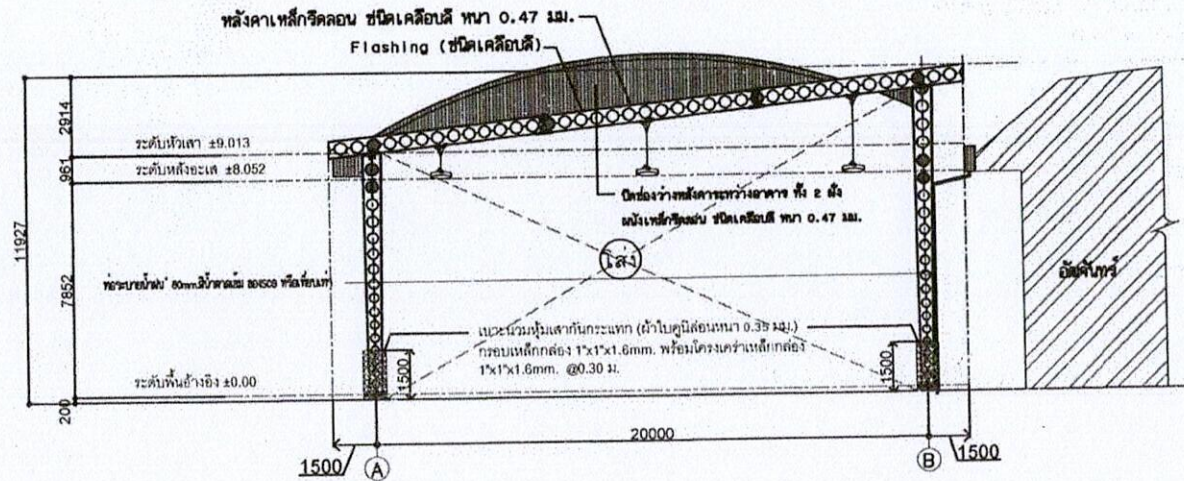
รูปด้านทิศตะวันออกและทิศตะวันตก อาคารหลังที่ 2
